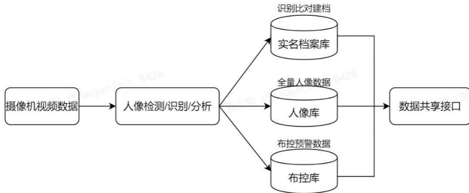
图 A.2 系统数据流程图
