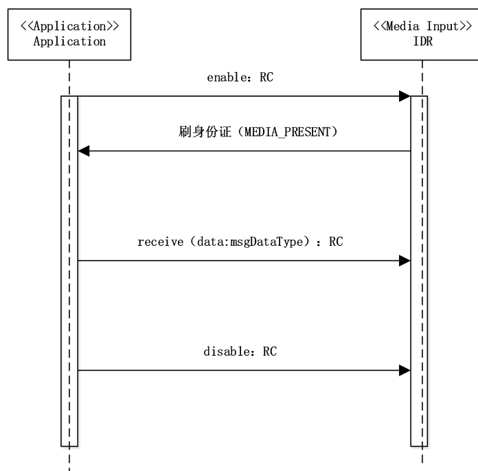
图 21 身份证阅读器的典型序列图
