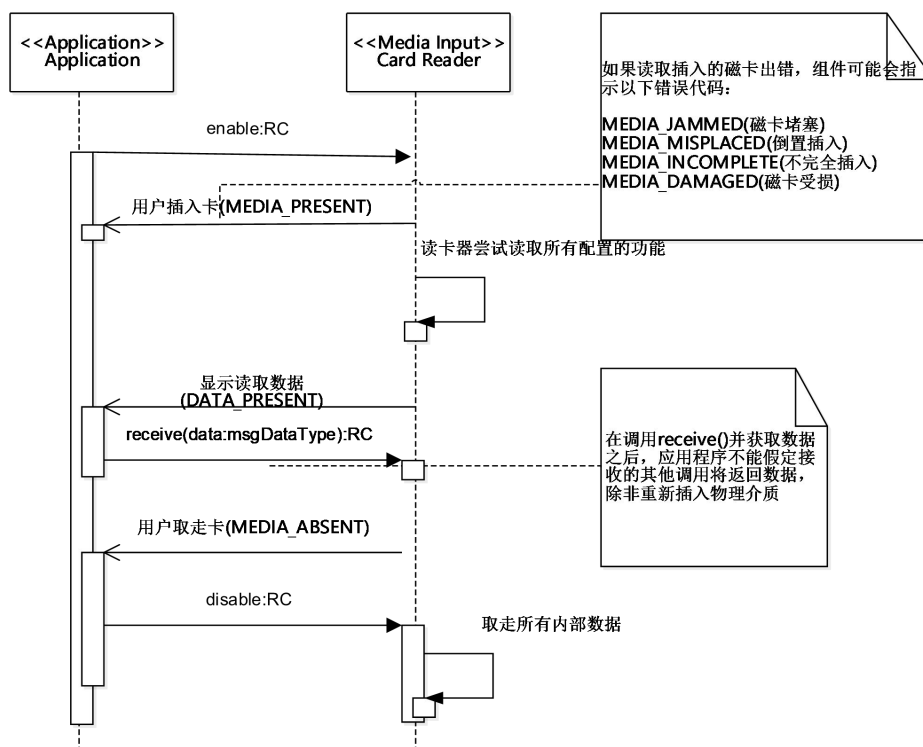
图 10 插卡式磁卡读卡器的典型序列图
