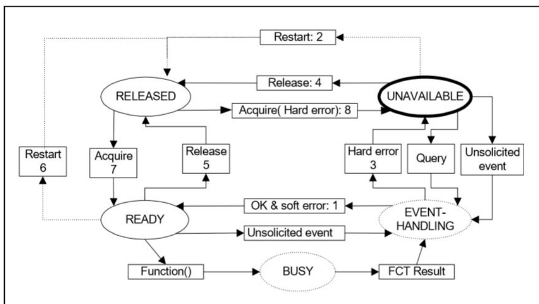
图 4 设备组件状态图（航司应用视图）
