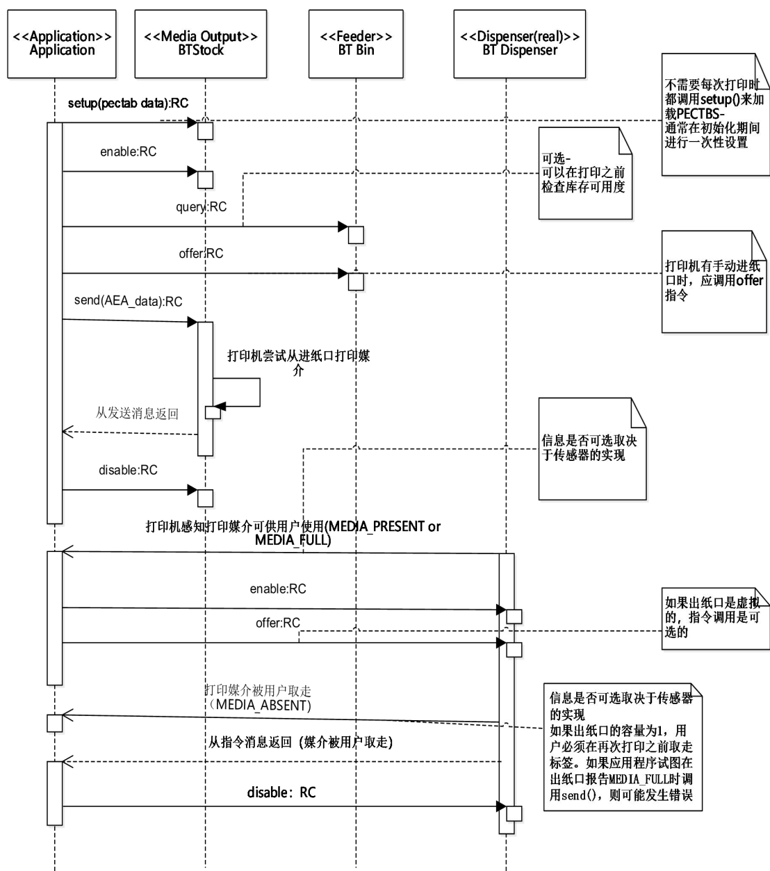
图 8 行李条打印机的典型序列图
