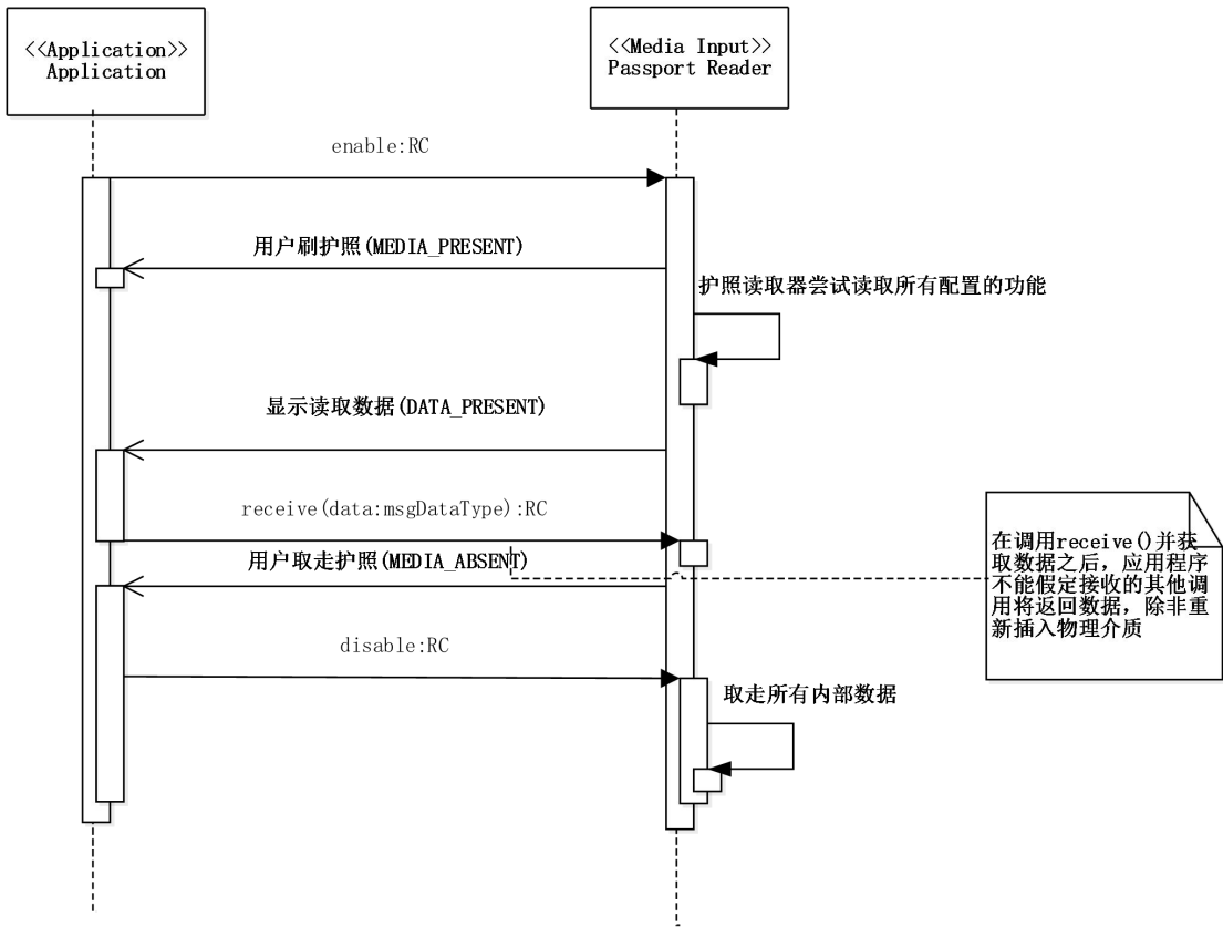
图 15 刷卡阅读器上读取护照的典型序列图
