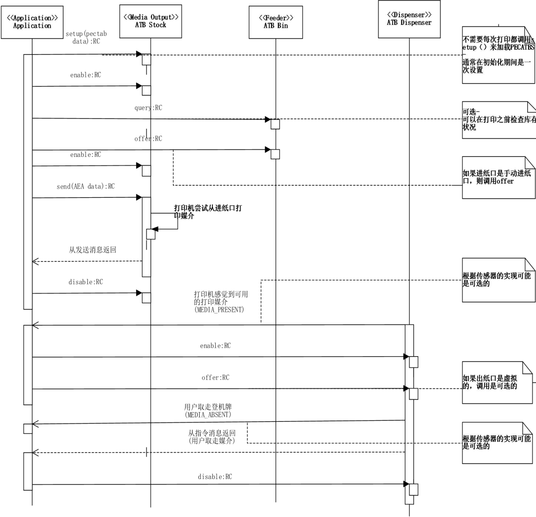
图 6 ATB 打印机的典型序列图
